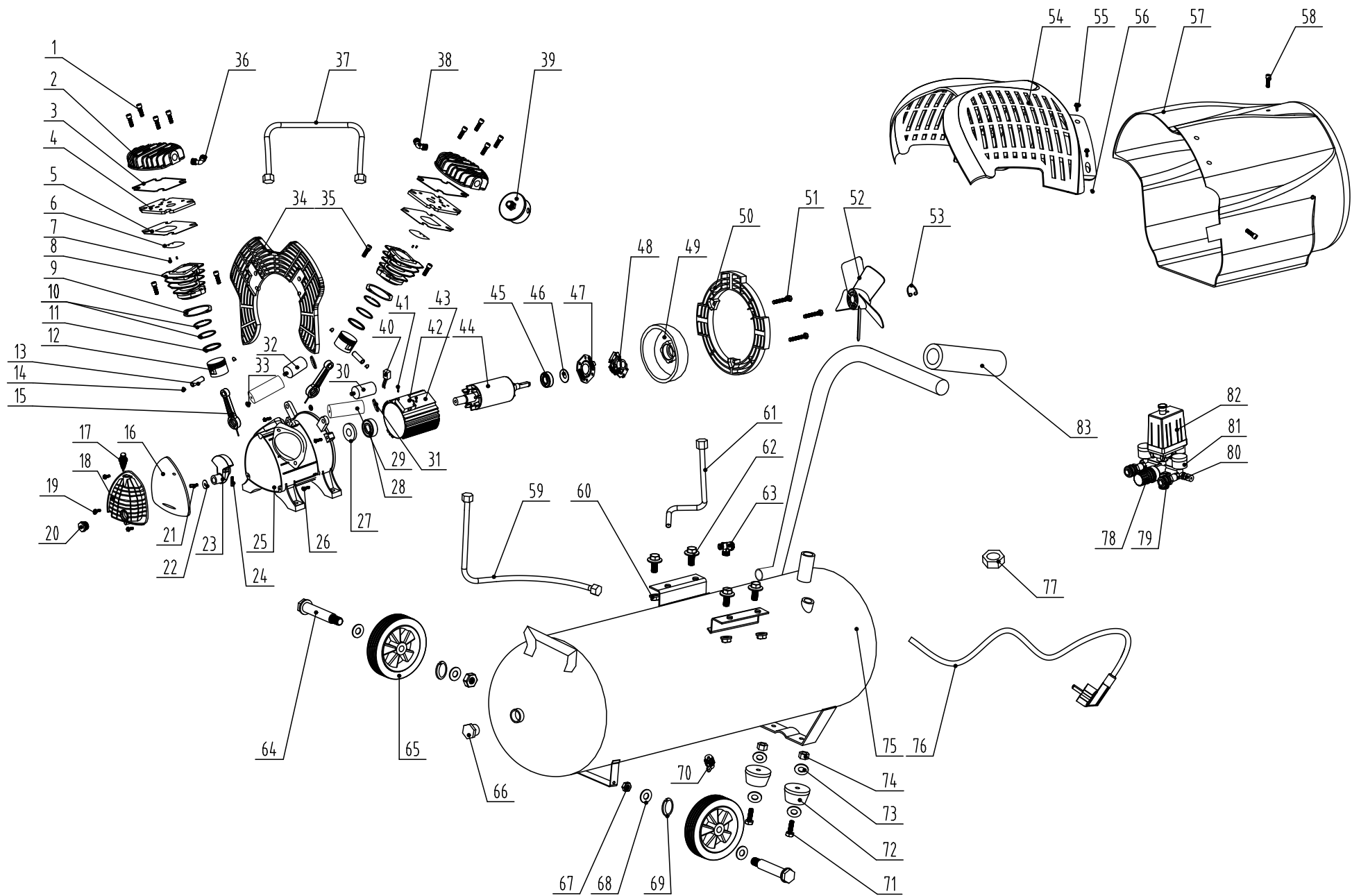
51.02-K-2200 kompresor 2.2 kW, nádoba 50L
