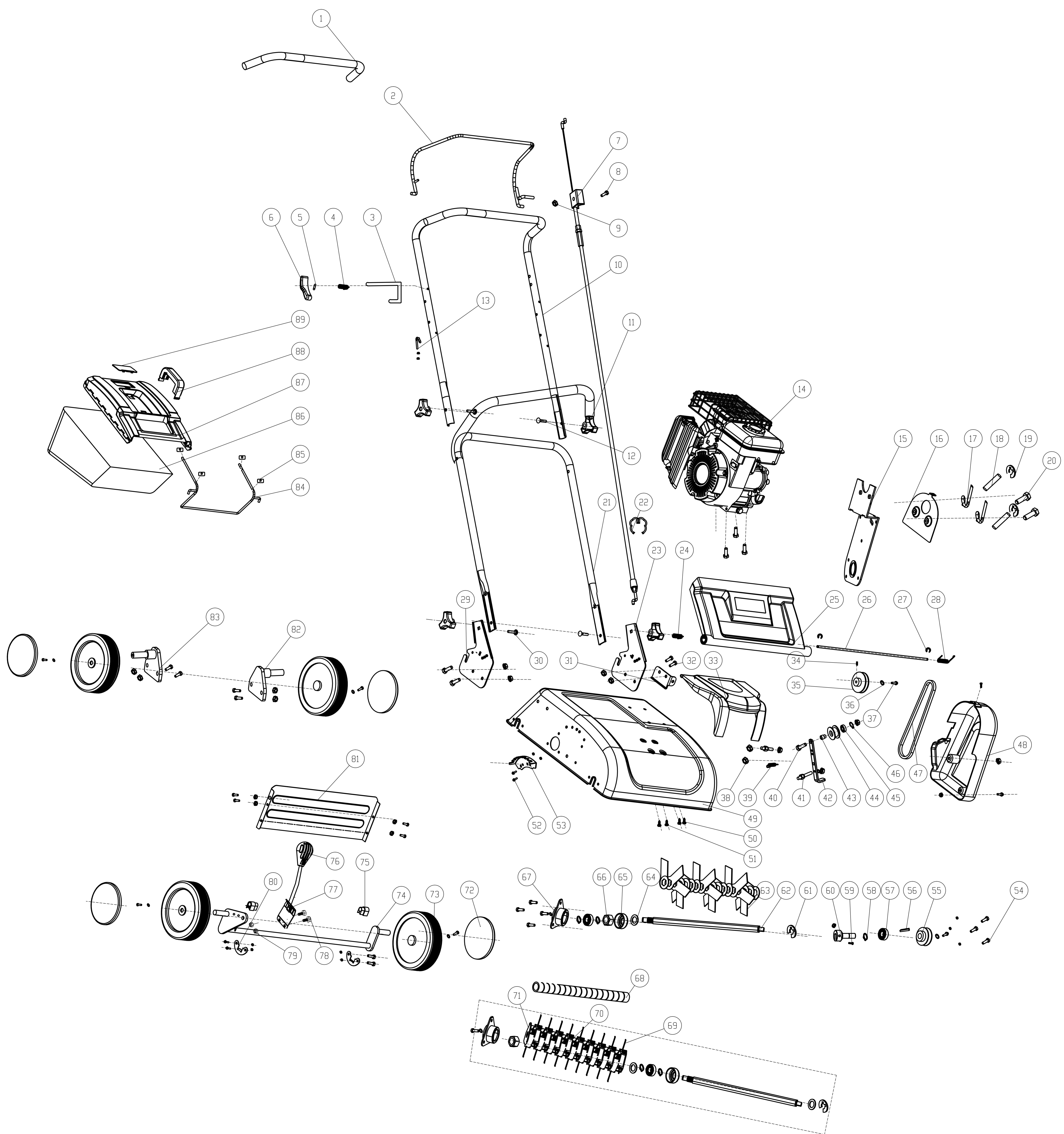
51.06-VB-380 vertikutátor benzínový a provzdušňovač trávníku 2v1 4,3 kW
